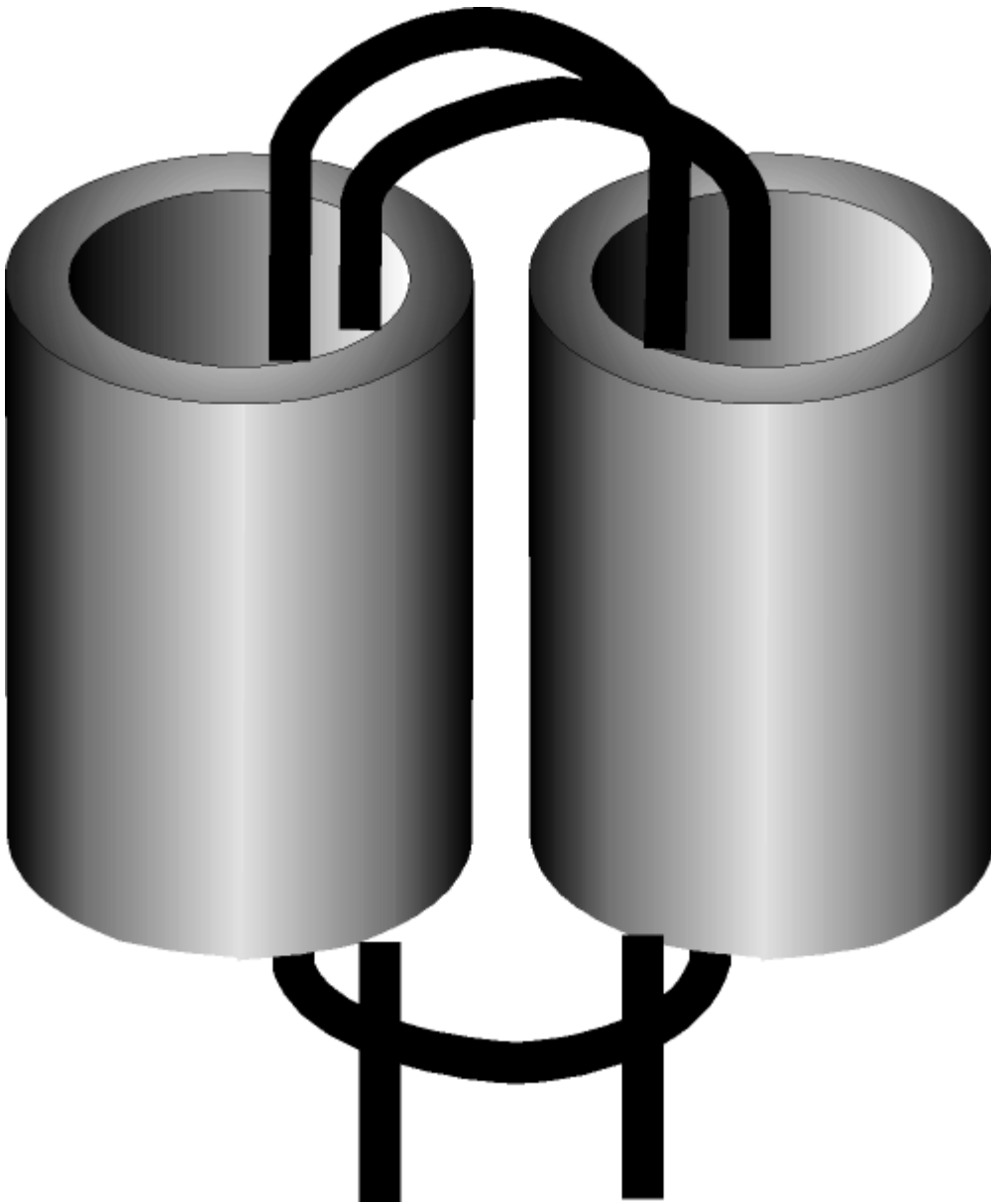
Vue sur un enroulement avec deux tubes ferrite juxtaposés
